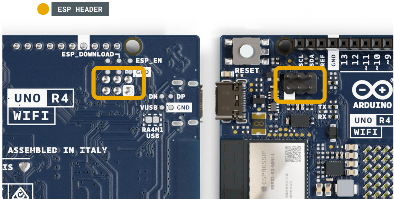
ESP引脚
